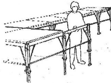
Ainsi de suite jusqu'à l'obtention de la base complète
